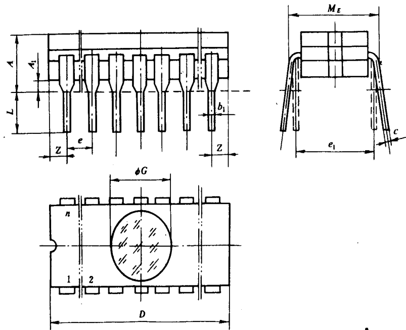
图 5-1-1 跨度为 10.16mm 带光窗封装外形图
