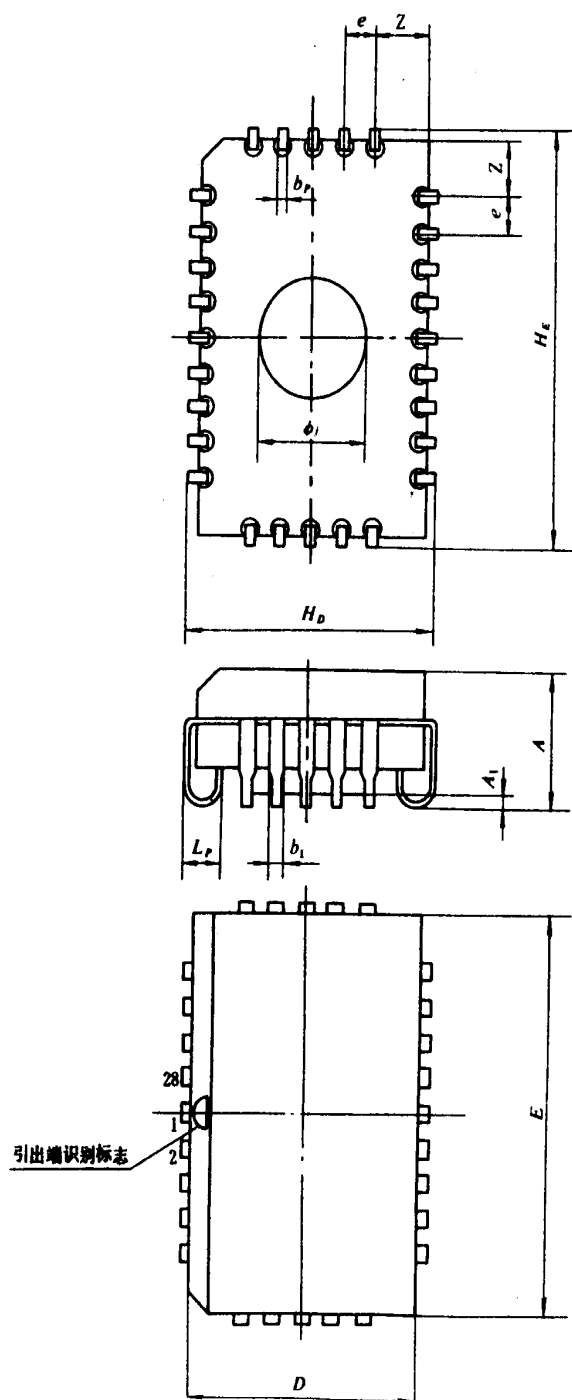
图 3-5-5 长方形塑料片式载体封装外形图
