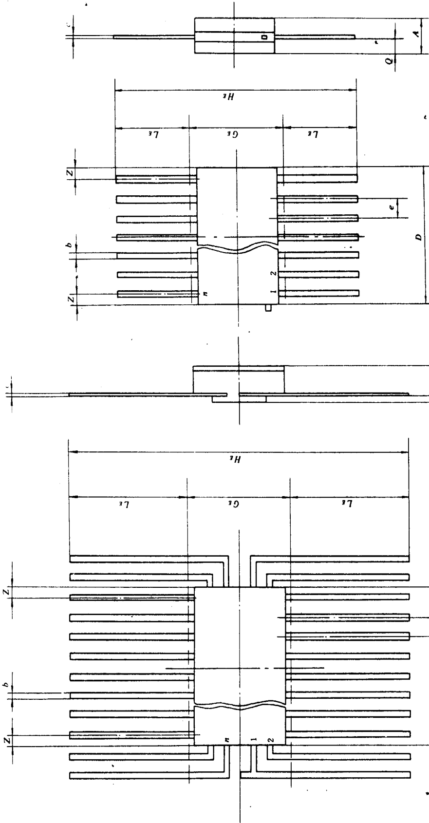
图 2-4-1 引线两面引出陶瓷熔封扁平封装外形图
