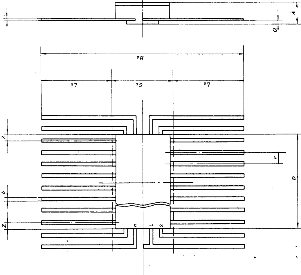
图 2-3-3 长引线四边布线两面引出陶瓷扁平封装外形图
