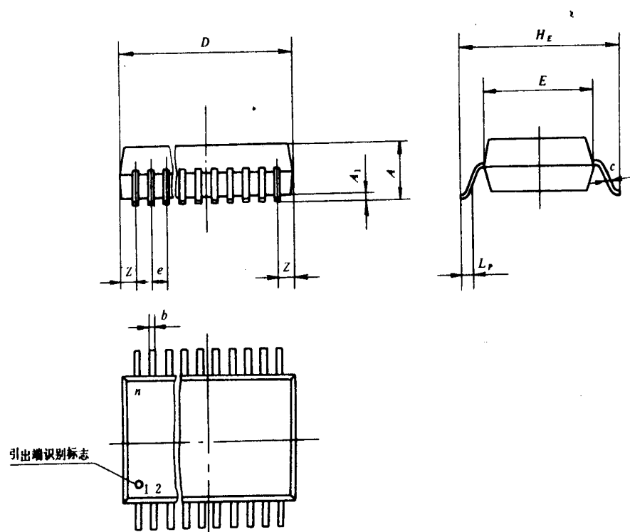
图 3-8-1 跨度为 7.62mm 缩小型小外形塑料封装外形图
