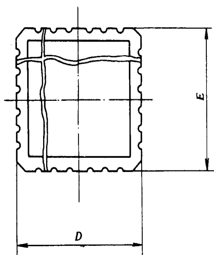
图 2-5-3 间距为 1.00mm 正方形无引线陶瓷片式载体封装外形图
