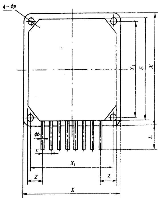
图 4-2-3 引线单面引出方形金属扁平封装外形图
