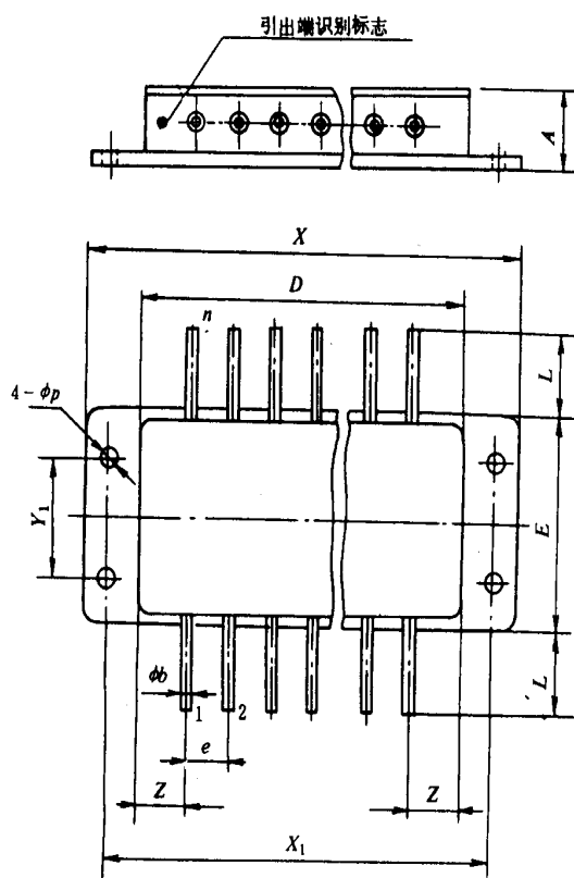
图 4-2-1 引线正面引出矩形金属扁平封装外形图
