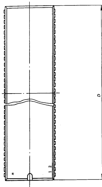
图 3-7-4 跨度为 19.05mm 缩小型塑料双列封装外形图
