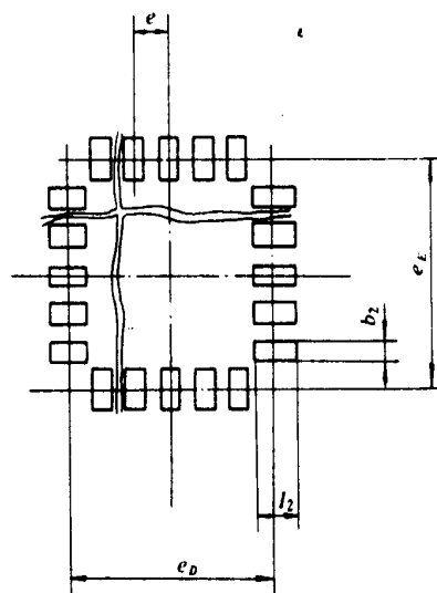
图 2-5-2 引出端焊接区图形
