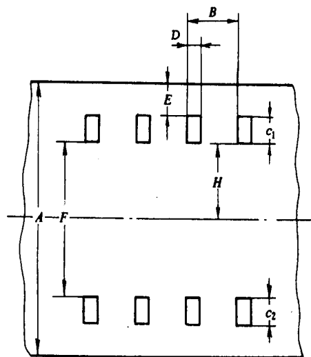
图 5-3-7 载带自动焊接封装部位尺寸图
