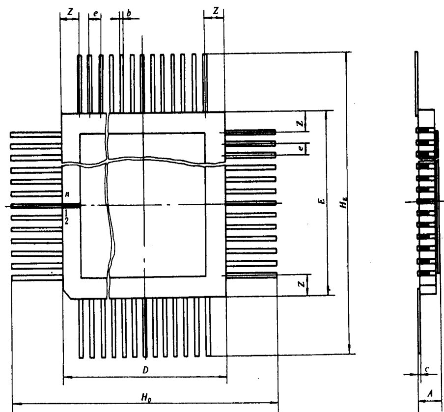
图 2-6-2 间距为 1.00mm 陶瓷四面引线扁平封装外形图
