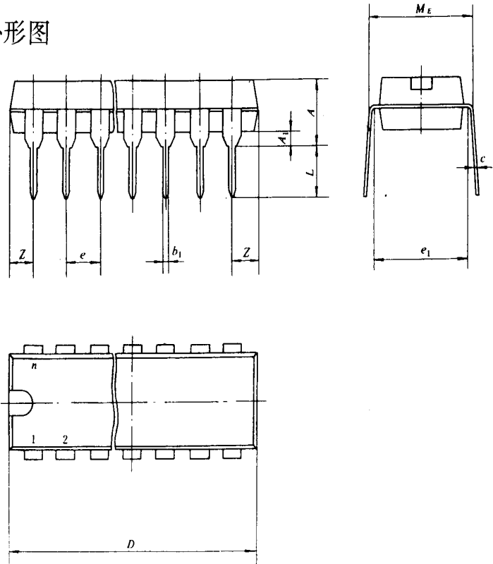
图 3-1-1 跨度为 7.62mm 塑料双列封装外形图
