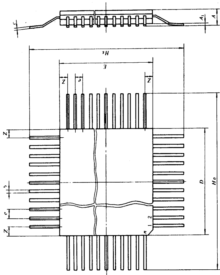
图 2-5-13 翼形引线陶瓷片式载体封装外形图
