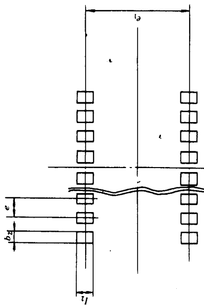
图 3-2-4 引出端焊接区图形
