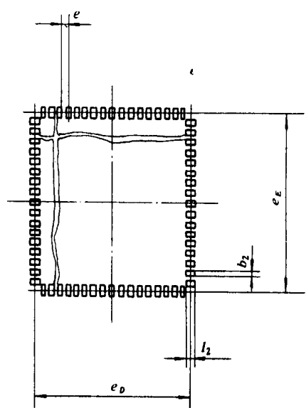
图 2-5-8 引出端焊接区图形
