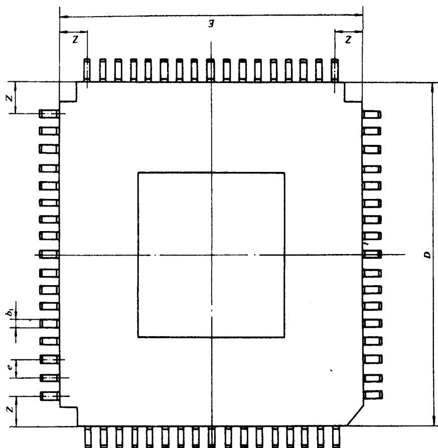
图 2-5-11 反“J”形引线陶瓷瓷片式载体封装外形图
