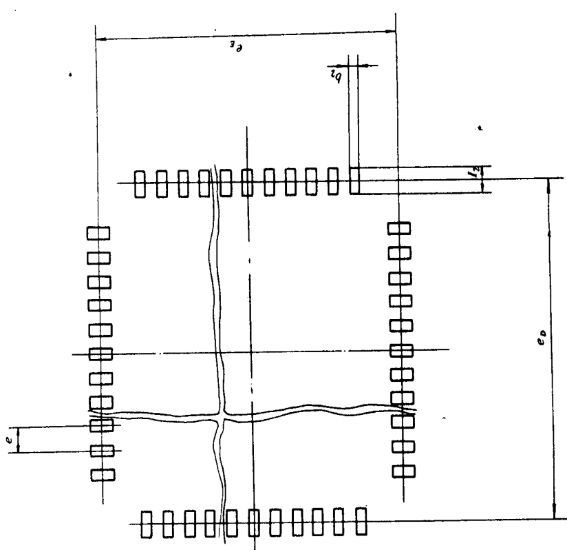
图 2-5-14 引出端焊接区图形
