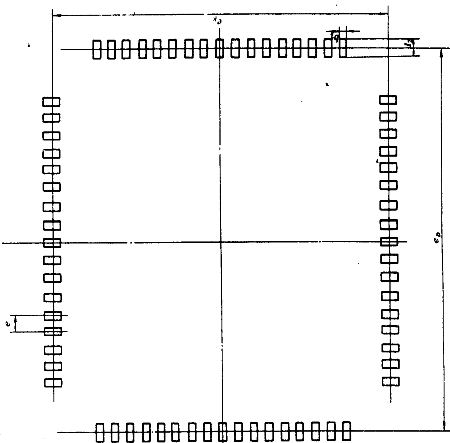
图 2-5-12 引出端焊接区图形
