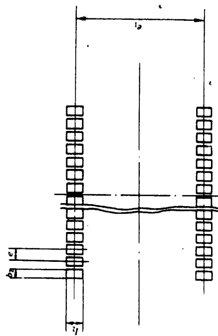
图 3-8-4 引出端焊接区图形
