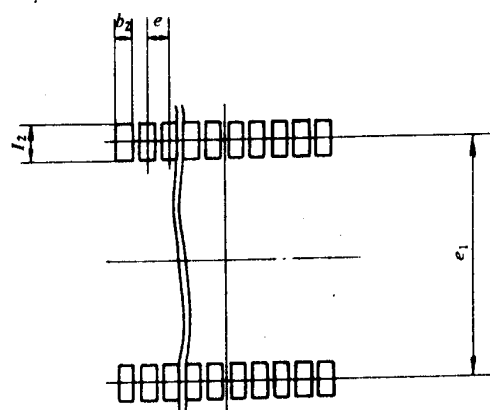
图 3-8-2 引出端焊接区图形
